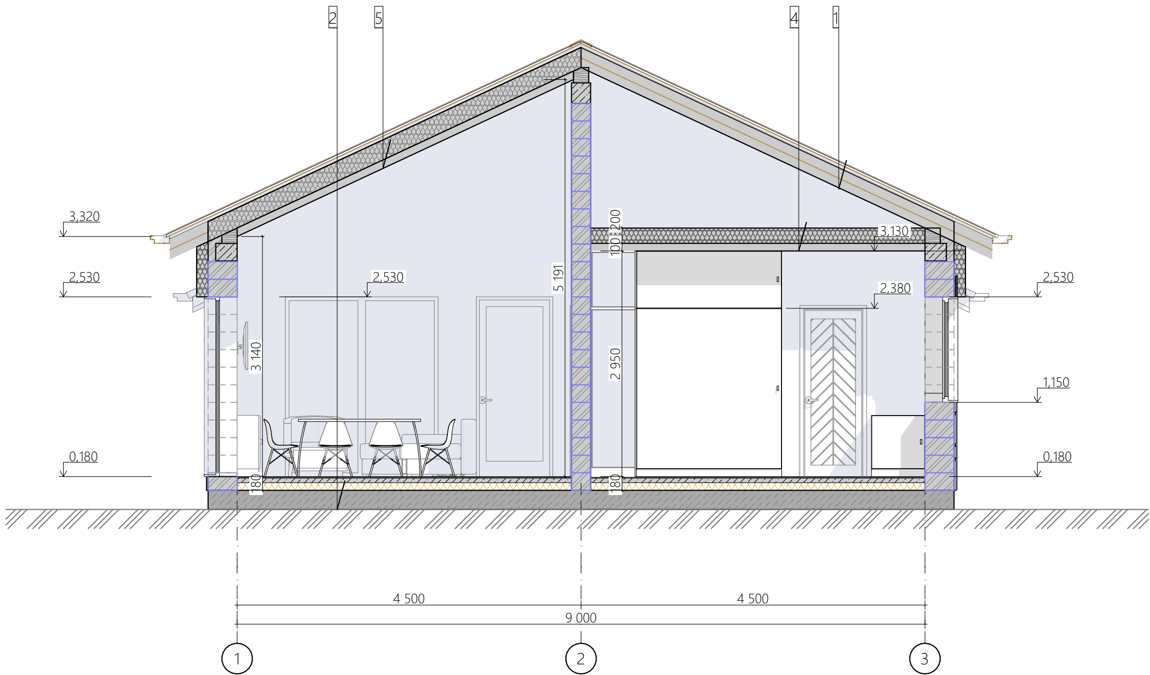
Разрез 2-2
